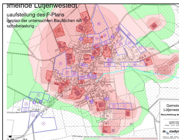
Abbildung 21 - Geruchsimmissionsprognose 2020
